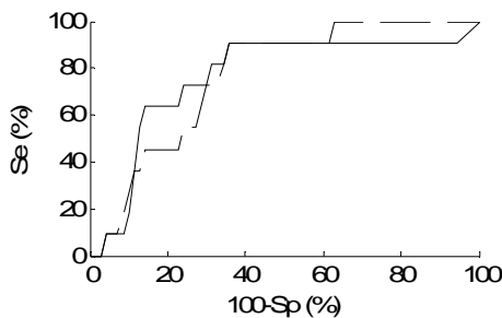
Figura 3. Curvas ROC para r_{\text{DAP}} (línea discontinua) y r_{\text{DAP}}^a (línea continua).
