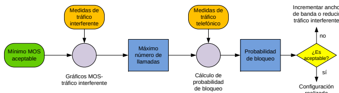
Fig. 18. Diagrama de flujo para configurar el sistema CAC
