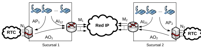
Fig. 5. Líneas de gateway compartidas
