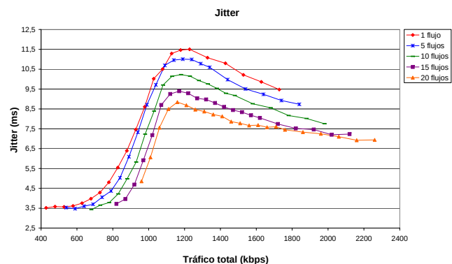
Fig. 16. Jitter en función del tráfico total
