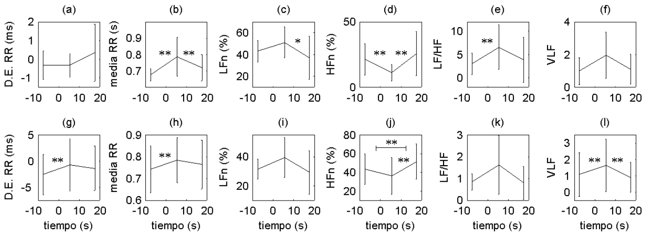
Figura 2. Test One way ANOVA para medidas repetidas. Apnéicos (a-f), No-apnéicos (g-l). * p < 0.05 ** p < 0.01
