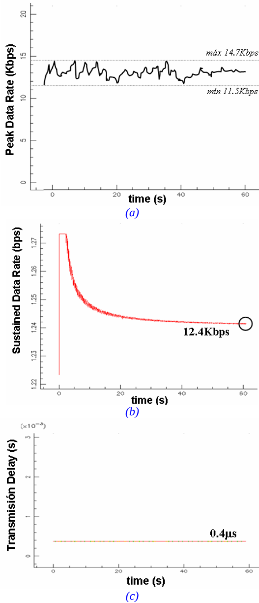
Fig. 4. QoS3 Básico aplicado a servicio RT de audio. (a) PDR (bps) (b) SDR (bps) (c) \tau_{c,i}^l (s)
