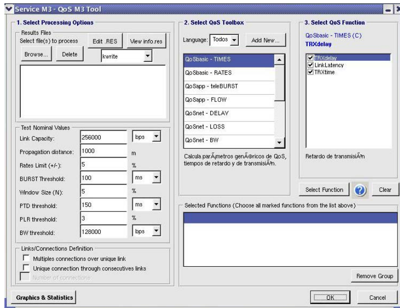
Fig. 1. Captura gráfica de la herramienta QoSM3.
