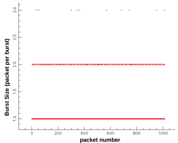
Fig. 10: Tamaño instantáneo de la ráfaga.
