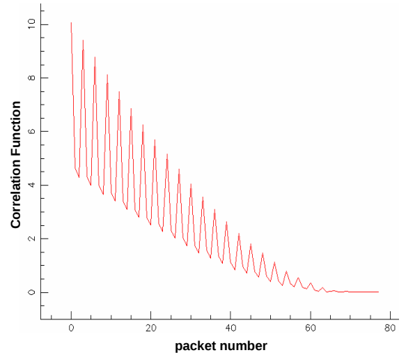
Fig. 8. Función de autocorrelación para el servicio RT de vídeo Netmeeting.
