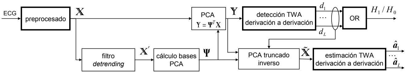
Figura 2. Diagrama de bloques del esquema multiderivacional. Los bloques en negrita son los que se usan en el esquema monoderivacional, en el que \mathbf{Y} = \mathbf{X} = \tilde{\mathbf{X}} .
