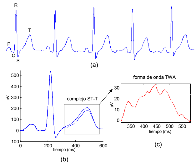
Figura 1. (a) Señal ECG con TWA visibles. (b) Superposición de dos latidos consecutivos. (c) Forma de onda de las TWA.
