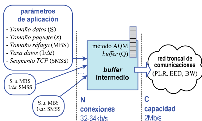
Figura 1. Esquema genérico de evaluación
