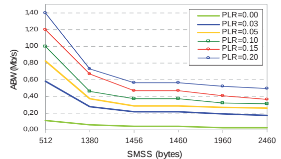
Figura 5. Evolución de ABW según SMSS con PLR variable
