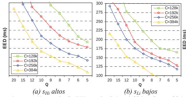
Figura 6. Variación de EED según Q ( r_1=64\text{kb/s} y C variable)
