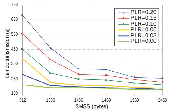
Figura 3. Evolución de T según SMSS con PLR variable
