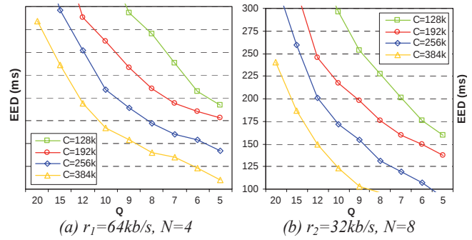
Figura 7. Valores de EED según r_1 ( s_{Hi} altos y C variable)
